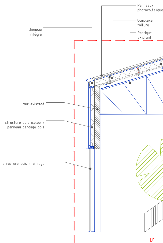
Détails constructifs de la structure
